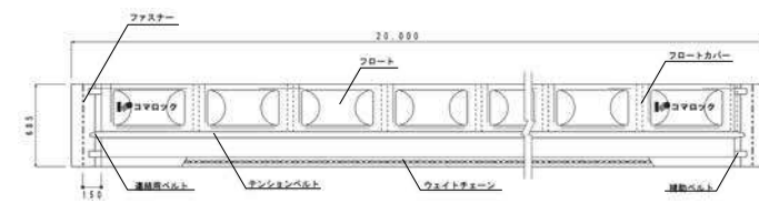
防舷材取付工事時設置状況
